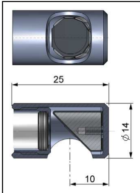
Rechtwinkel-Spiegelvorsatz Ermöglicht Messungen im 90°-Winkel zur Sensor- achse [ACCTRAM].
