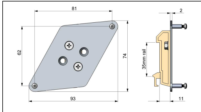
Tragschienenmontageplatte für Elektronik-Box [ACCTRAIL]
