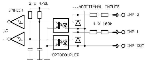
Abb. 3: Schaltbild Eingang
