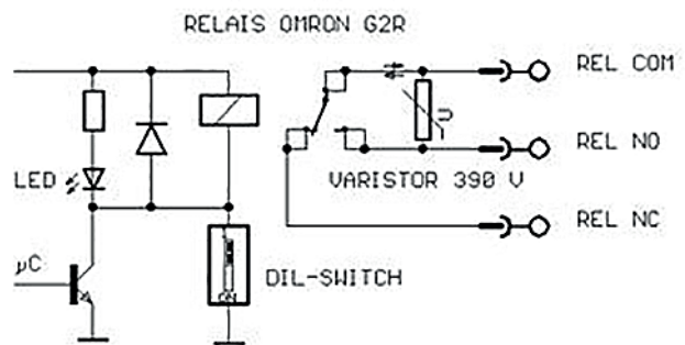
Abb. 4: Schaltbild Ausgang
